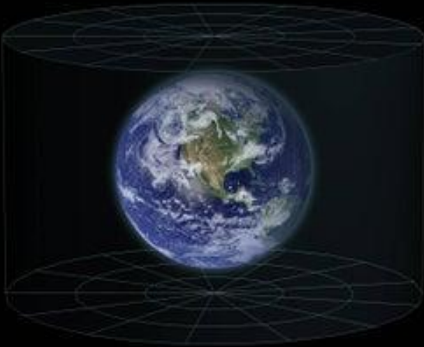
Earth
